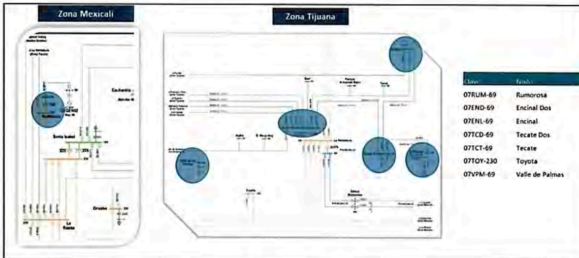
Figura 3. Ubicación de los Centros de Carga del Acueducto Río Colorado - Tijuana
