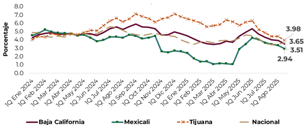
Grafica 13. Crecimiento de la inflación quincenal interanual de Baja California, Mexicali Tijuana y nacional. Primera quincena de enero 2024 a la segunda quincena de agosto 2025.
